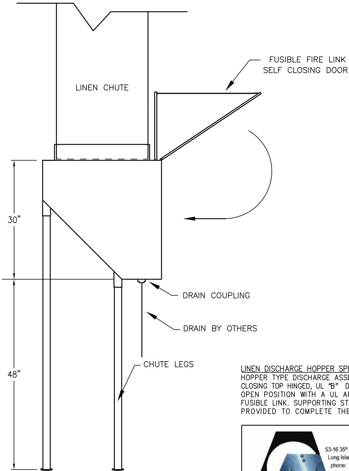
HOPPER TYPE CLOSING GATE N.T.S.
