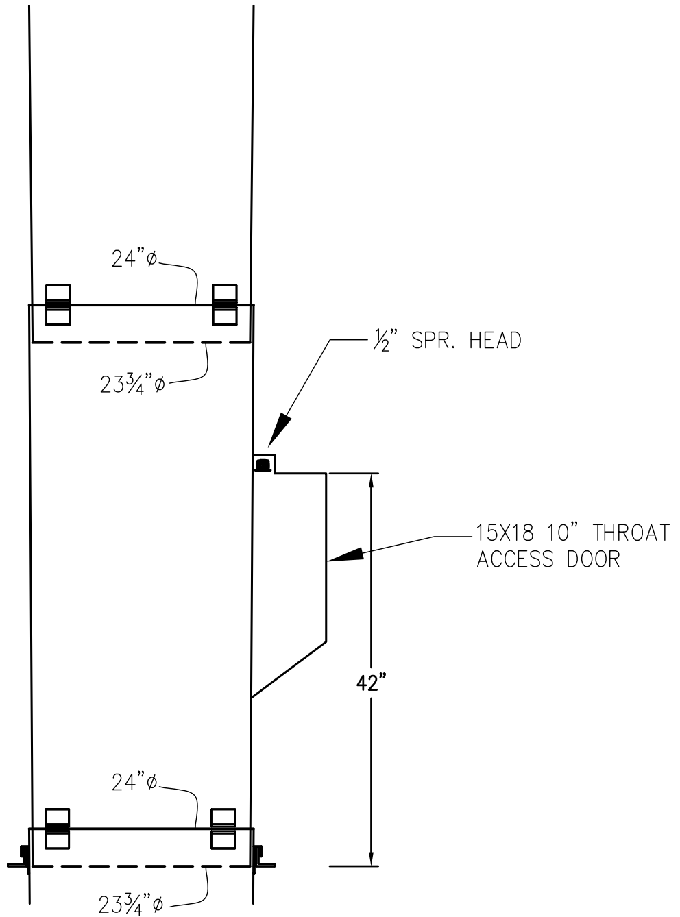
TRASH CHUTE INTAKE N.T.S.
