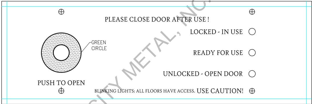
BEZEL PLATE DETAIL FOR ISD TRASH DOOR
